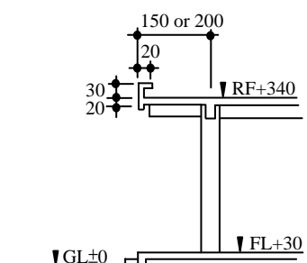
●高程示意圖
